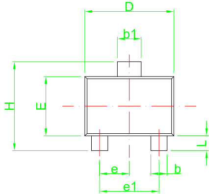
TOP SIDE
