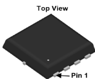
PDFN3x3-8L
