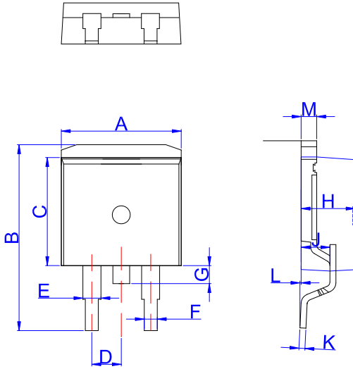
TO-263
