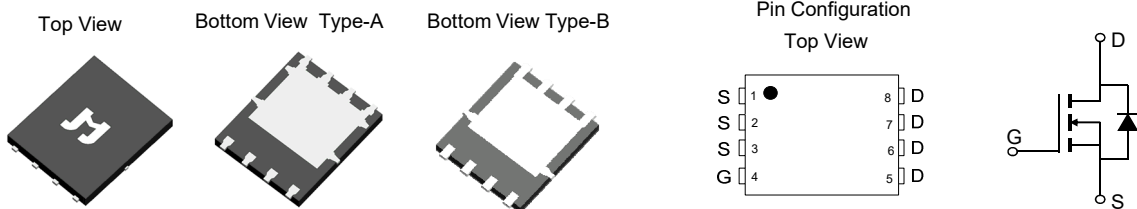
PDFN5x6-8L
