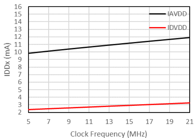
图 7-25 供电电流 vs 时钟频率
