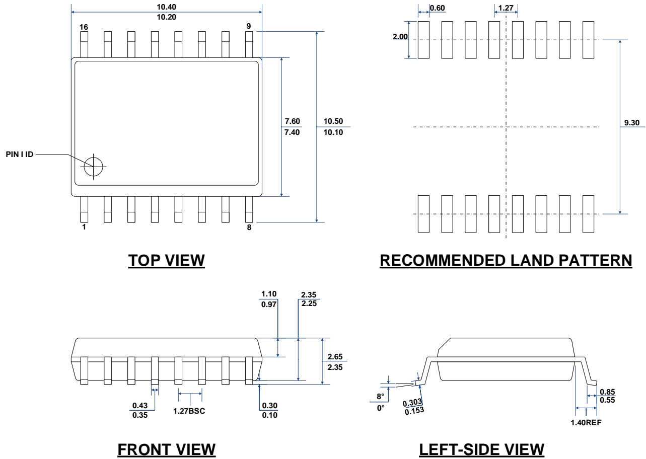
图 10-1 SOIC16 宽体封装外形尺寸图
