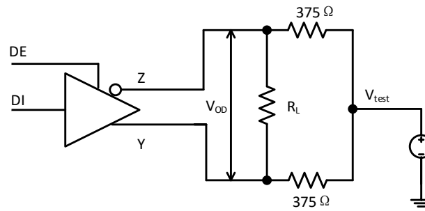
图 8-1. 驱动器差分输出电压 @ 共模负载
