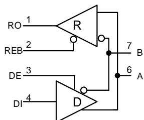
CA-IF4805H 简化框图
